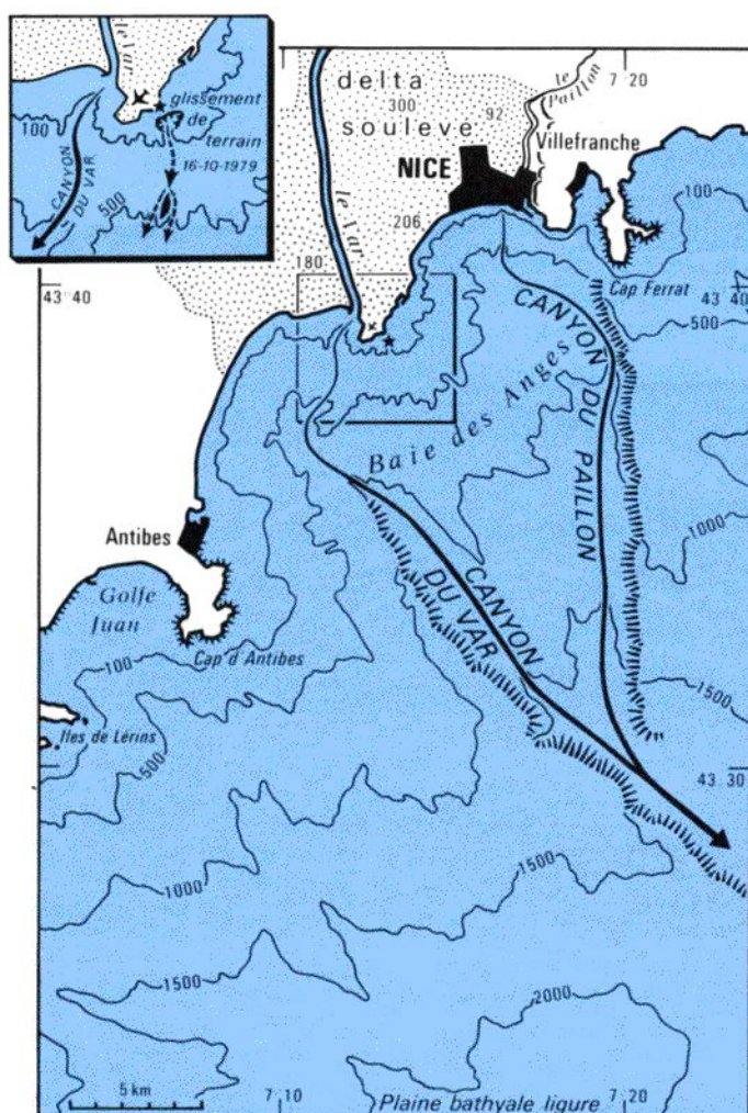
1. Prodélta du Var: croquis de localisation Prodelta of Var River: location sketch
