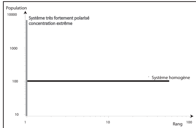
Figure 8: distributions rang-taille de systèmes de villes de référence
